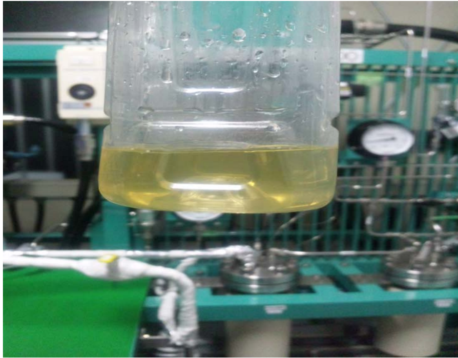
B T LプラントのF T合成油（ブドウ、桃木のチップからバイオ軽油）
